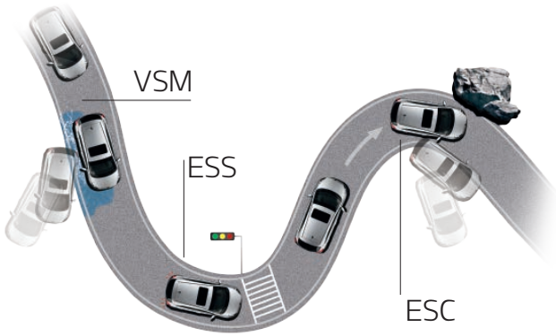
Elektroniczny układ stabilizacji toru jazdy (ESC) W przypadku gwałtownego hamowania układ ESC steruje siłą hamowania każdego koła z osobna. W ten sposób pomaga kierowcy zachować panowanie nad pojazdem.
