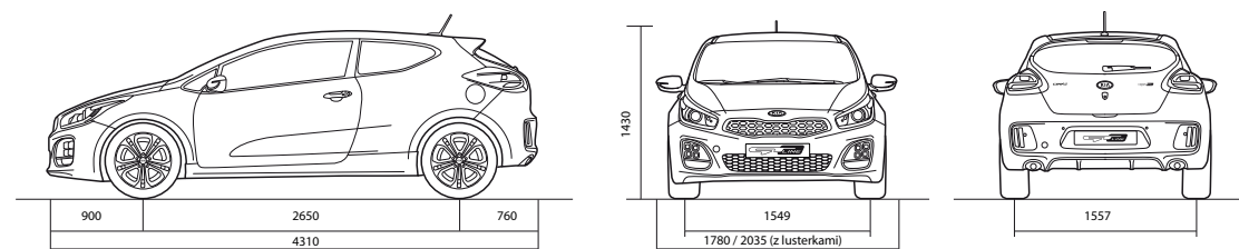
Kia pro_ceed GT Line — wymiary zewnętrzne (mm)
