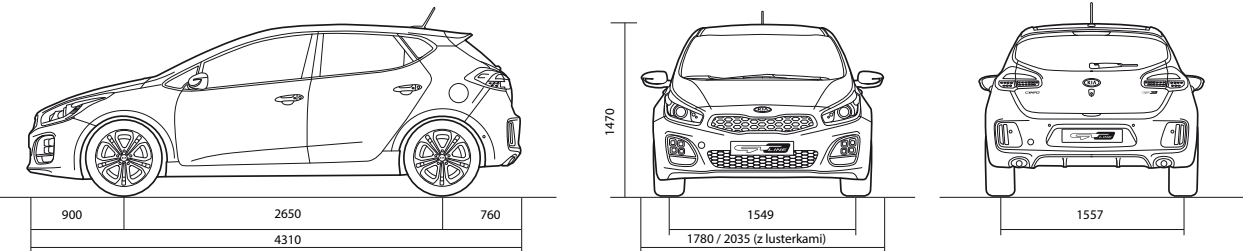
Kia cee'd 5-drzwiowa GT Line — wymiary zewnętrzne (mm)
