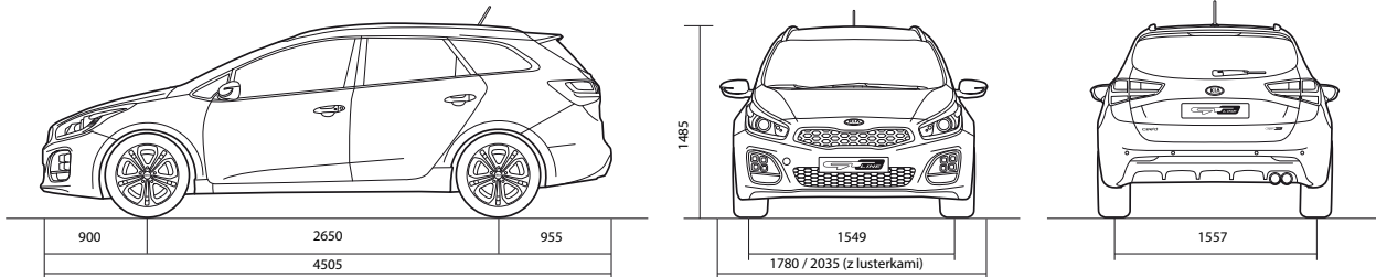
Kia cee'd kombi GT Line — wymiary zewnętrzne (mm)
