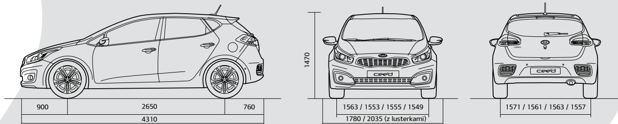
Kia cee'd 5-drzwiowa — wymiary zewnętrzne (mm)
