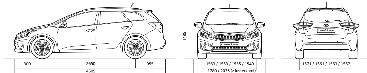
Kia cee'd kombi — wymiary zewnętrzne (mm)
